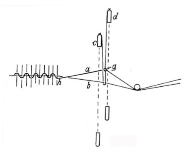
Abb. 146: Grundprinzip Drehergewebe mit Glasaugenlitzen
