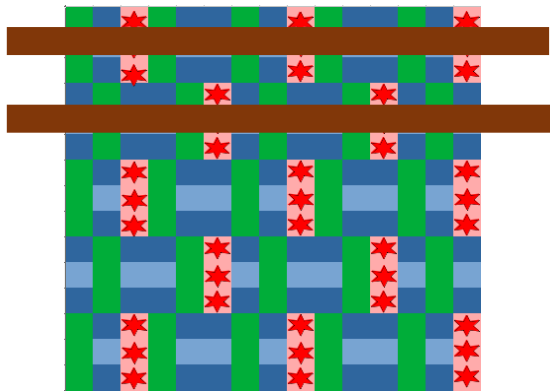
Abb. 158: Patrone der Samtbindung mit Ruten (braun) und aufgeschnittener aufgeschnittener Florkette (rote Sterne)
