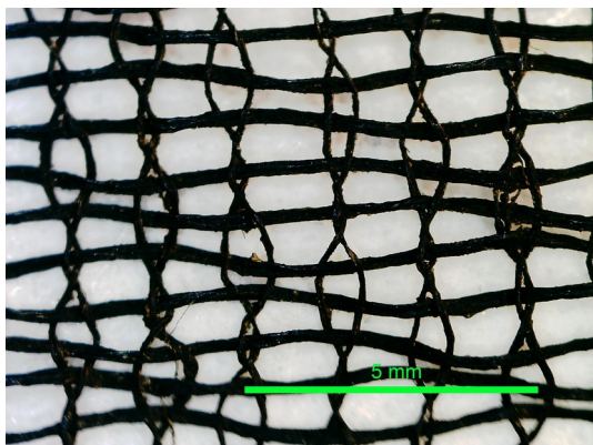
Abb. 136: Makroaufnahme Gaze- bzw. Dreherbindung, Besatz und Aufputz
