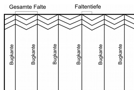
Abb. 186: Technische Darstellung der Falten
