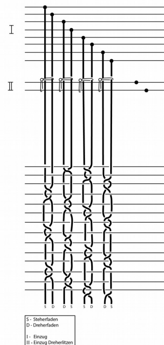
Abb. 149: Schematische Darstellung der Gaze mit Einzug
