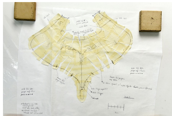
Abb. 199: Abgenommener Schnitt, Haube B, Maßstab 1:1
