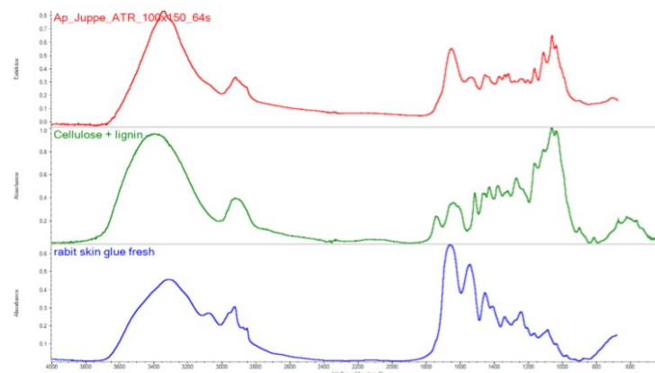
Abb. 181: Ergebnisse der FTIR-Analyse zur Appretur der Juppe. Die rote Linie zeigt das Spektrum der Appretur von Juppe. Die blaue Linie das Spektrum von Hasenhautleim als Referenzmaterial
