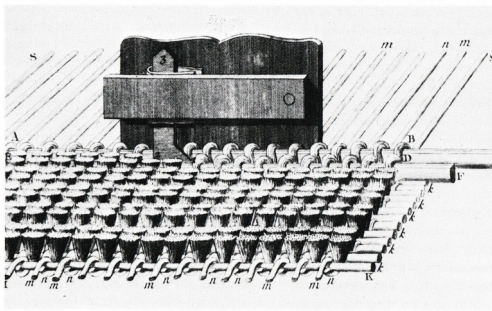
Abb. 154: Herstellungstechnik eines Samtes
